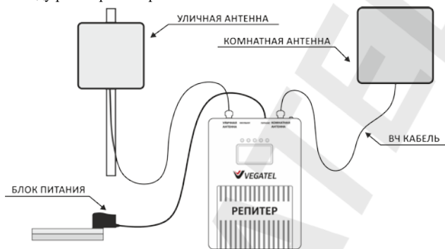
СХЕМА ПОДКЛЮЧЕНИЯ РЕПИТЕРА
